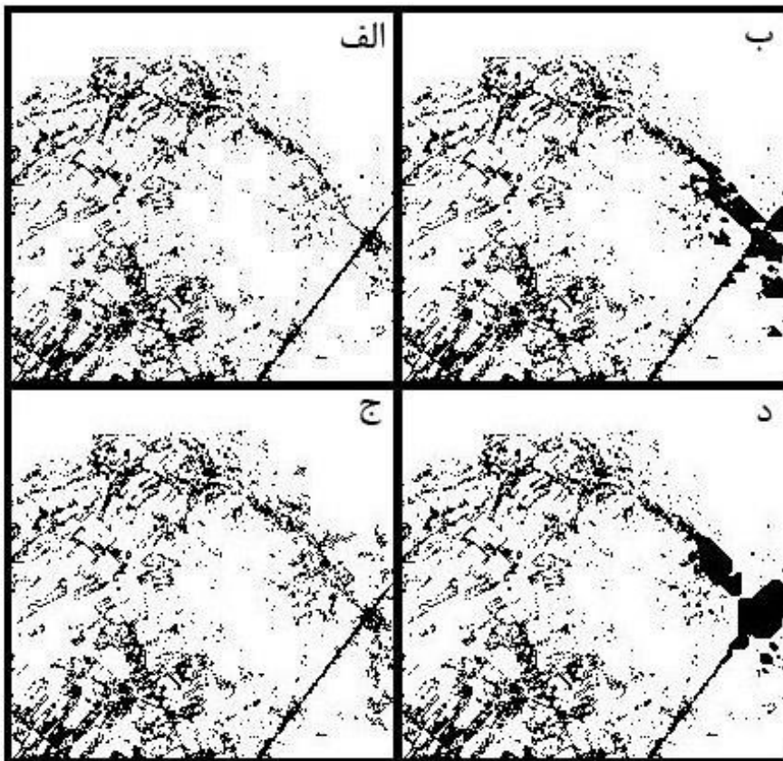
شکل ۵. تفاوت نتایج شبیه‌سازی ناشی از تغییر قانون انتقال سلول‌های خودکار طی بهینه‌یابی با الگوریتم گرگ خاکستری در سطح محلی (الف تصویر پایه؛ ب و ج و د نقشه شبیه‌سازی شده به ترتیب با ۱٫۵، ۳ و ۶ درصد رشد شهری)
