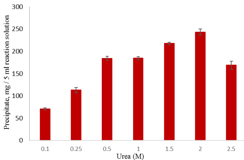
شکل ۲- مقایسه مقدار رسوبات در غلظت‌های مختلف اوره.
