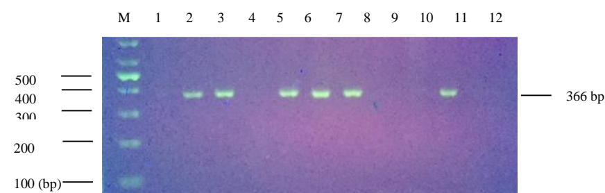
شکل ۲- محصول AS-PCR پلی مورفسم rs632478 A/C بر روی ژل آگارز ۲ درصد که نشان دهنده تکثیر آلل C مورد نظر با استفاده از پرایمرهای Forward2 و Reverse است. M معرف مارکر مولکولی و چاهک‌های ۲، ۳، ۵، ۶، ۷ و ۱۰ نشان دهنده قطعه تکثیر شده هستند.
