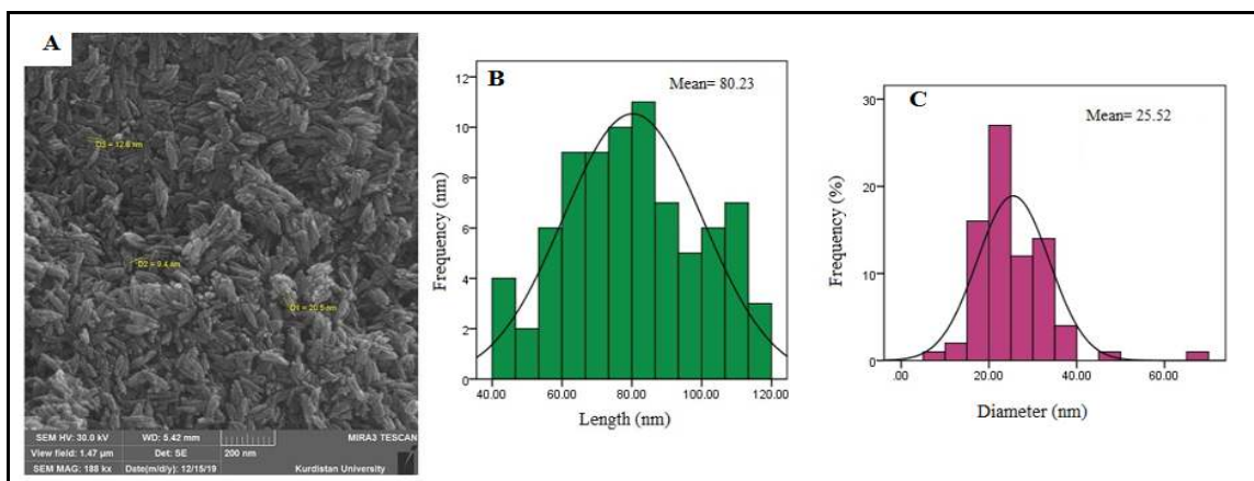
شکل ۷- تصاویر حاصل از FESEM. A. تصاویر حاصل از FESEM. B و C. هیستوگرام توزیع اندازه نانوذرات برون سلولی مگنتیت تولیدی تحت استراتژی عصاره عاری از سلول.
