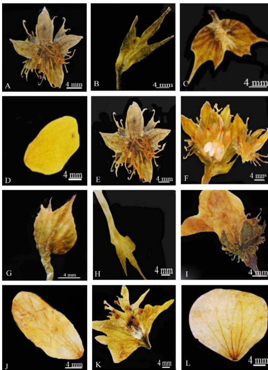
شکل ۲- ریخت‌شناسی گل در زیرطایفه Agrimoniinae . A-C. Agrimonia eupatoria subsp. eupatoria . D-G. A. eupatoria subsp. grandis . H-I. A. eupatoria subsp. asiatica . J-L. Aremonia agrimonioides . Fig. 2. Flower morphology in subtribe Agrimoniinae . A-C. Agrimonia eupatoria subsp. eupatoria . D-G. A. eupatoria subsp. grandis . H-I. A. eupatoria subsp. asiatica . J, K. Aremonia agrimonioides .
