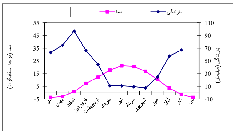
شکل ۳- منحنی باران دمایی ایستگاه جلفا. Fig. 3. Ombrothermic diagram of Jolfa station.
