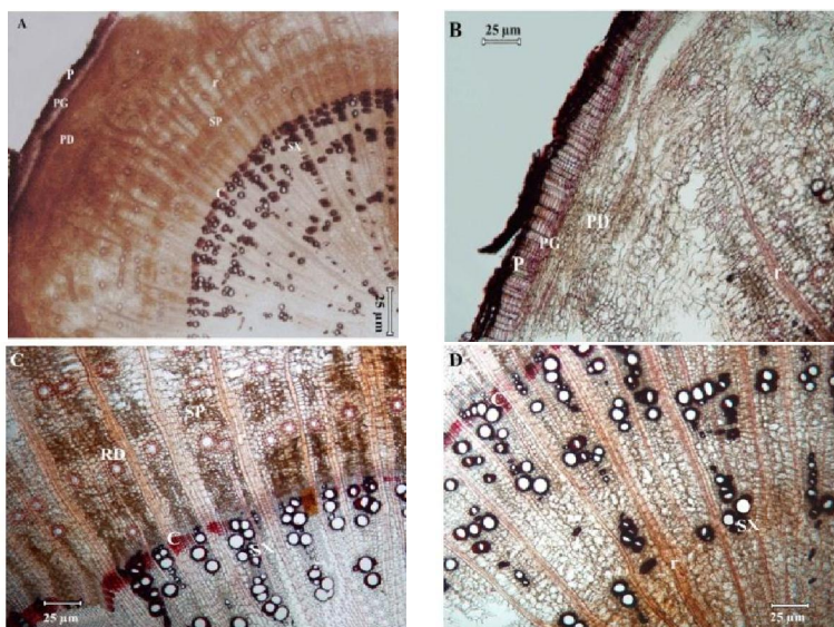
شکل ۶- برش عرضی ریشه کُهای سازوئی با میکروسکوپ نوری. A: بزرگ‌نمایی ۴X؛ B, C و D: بزرگ‌نمایی ۱۰X (P: فلم، PG: فلوژن، PD: فلودرم، PX: بافت آبکش ثانویه، SX: بافت چوب ثانویه، C: کامیوم، RD: مجرای رزین، R: پارانشیم رزین، T: اشعه آوندی).
