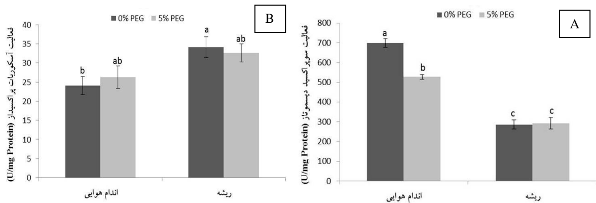
شکل ۱- اثر تنش خشکی بر A : میزان فعالیت سوپراکسید دیسموتاز و B : آسکوربات پراکسیداز در اندام هوایی و ریشه پونه معطر. (میانگین \pm SE). حروف یکسان مبین فقدان اختلاف معنی‌دار با استفاده از آزمون دانکن است ( p \leq 0.05 ).
