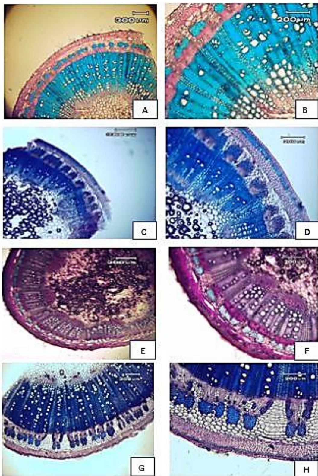
شکل ۴- ساختار برش عرضی ساقه در گونه های Alcea kurdica var. laxiflora : A-B، Alcea kurdica var. leiocarpa : C-D، Alcea rechingeri : E-F، Alcea sacsachanica : G-H
