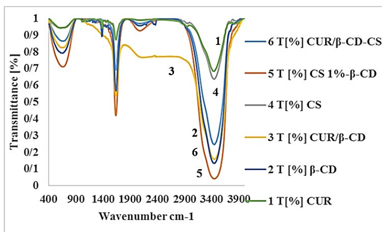
شکل ۳- طیف‌های FTIR برای CUR آزاد، \beta -CD خالص، کمپلکس CUR/ \beta -CD، CS خالص، \beta -CD-CS، و کمپلکس اصلاح شده CUR/ \beta -CD-CS. Figure 3. FTIR spectra for free CUR, pure \beta -CD, CUR/ \beta -CD complex, pure CS, \beta -CD-CS and CUR/ \beta -CD-CS modified complex.
