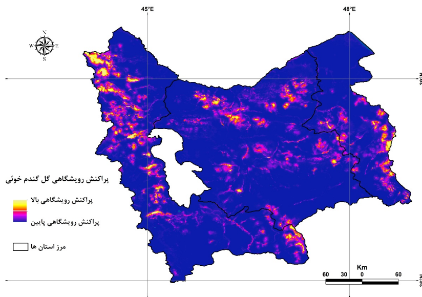
شکل ۴- نقشه اجماعی پراکنش رویشگاهی گل گندم خوئی در منطقه مورد مطالعه حاصل از میانگین وزنی شش مدل پراکنش رویشگاهی GAM، GLM، GBM و RF، MaxEnt، MARS. Figure 4. Ensemble habitat distribution map of Centaurea glastifolia in the study area result from mean-weighted of six habitat distribution model values i.e., GLM, GAM, MARS, MaxEnt, RF and GBM.
