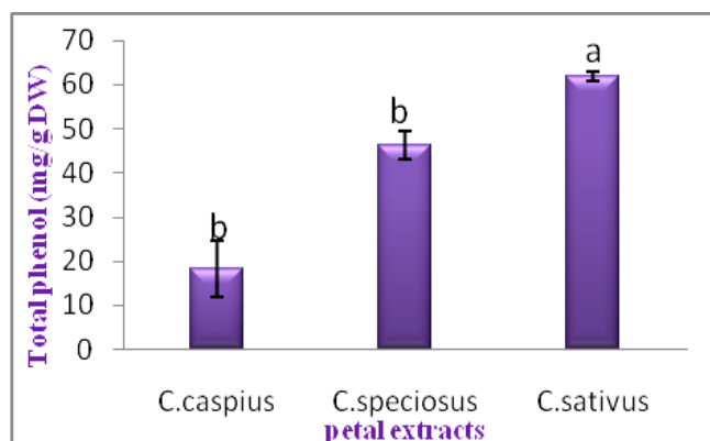
شکل ۲- میزان فنل کل در گلبرگ سه گونه مختلف زعفران. نتایج به صورت میانگین \pm انحراف معیار ارائه شده است ( P \leq 0.05 ). Fig. 2. The total phenol contents of crocus petals of three different species. Data shown as mean \pm S.E. ( P \leq 0.05 ).
