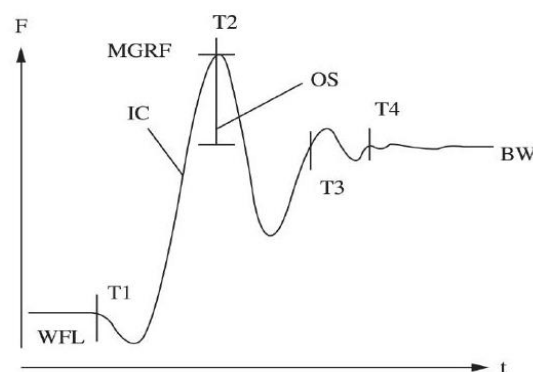
شکل ۱. نمودار مراحل حرکت نشست و برخاست به ۳ مرحله تقسیم‌بندی شده است. مرحله آماده‌سازی (T1-T2) مرحله برخاستن (T2-T3) مرحله ثابت (T3-T4) BW^2 وزن بدن، MGRF (حداکثر نیروی واکنش زمین)، OS ۳ (میزان خطا)، IC ۴ (شیب)، WFL ۵ (وزن کف پا/پا) مرحله استراحت، T1 ۶ (شروع حرکت)، T2 ۷ (نشسته)، T3 ۸ (برخاستن)، T4 ۹ (پایان حرکت) (۳۰)
