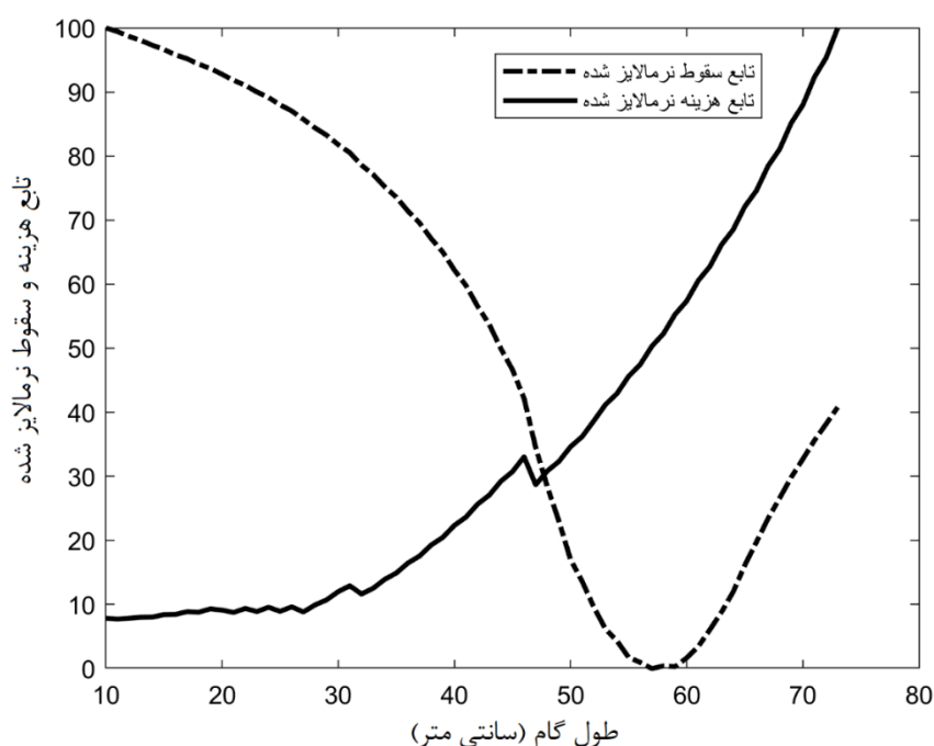
شکل ۷. تابع هزینه ازدست دادن تعادل و هزینه کل طبیعی شده در طول گام‌های متفاوت (۲۰-۷۳ سانتی متر)
