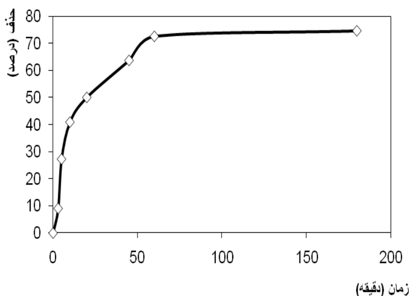
شکل ۴. منحنی درصد حذف فرمیک اسید بر حسب زمان (غلظت اولیه جذب شونده: ۰/۱ M، دما: ۲۹۵ K، مقدار جذب: ۳/۵ g)
