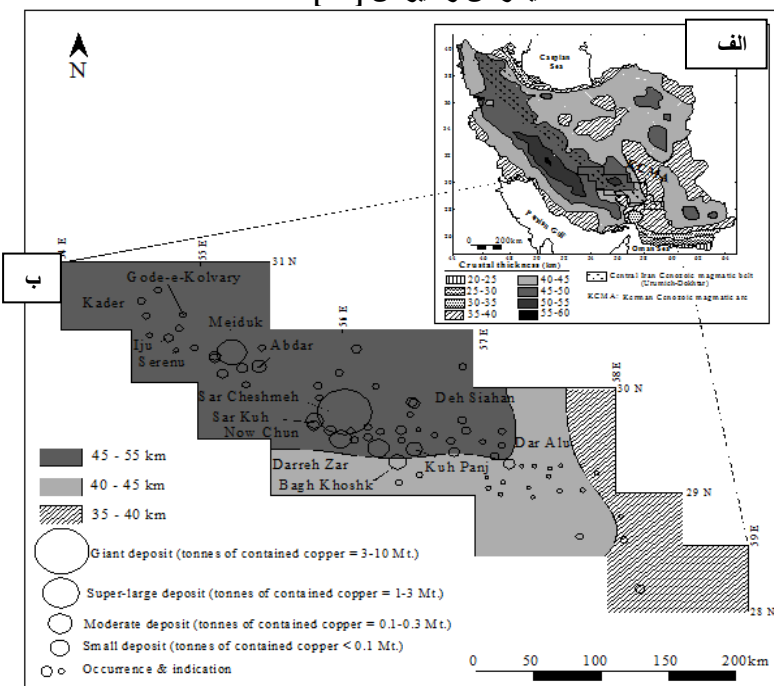
شکل ۲. الف) نقشه ساده شده ضخامت پوسته در گستره ایران بر پایه نقشه عمق امروزی موهو [۴۸] ب) نقشه تعبیرات ضخامت پوسته قاره‌ای در سراسر کمان ماگمایی سنوزوییک کرمان و تمرکز کانسارهای اصلی مس پورفیری در بخش‌های شمال غربی کمان که منطبق بر حداکثر ضخامت پوسته است [۱۷]
