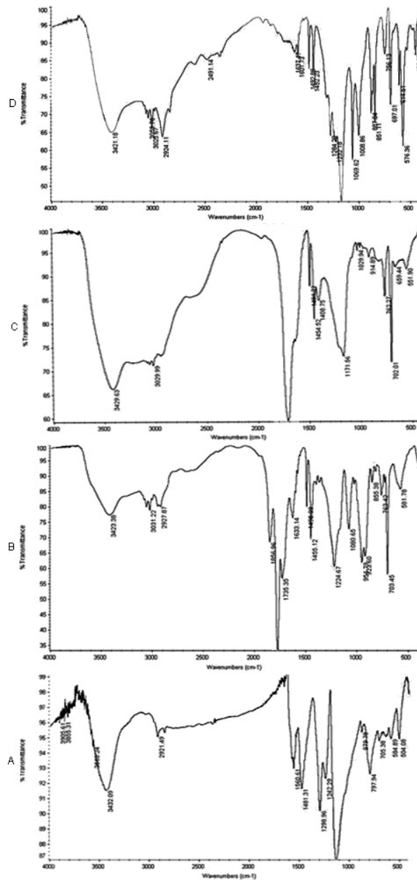
شکل ۴. طیف‌های IR مربوط به PSS (D)، PSMAC (C)، PSMA (B)، و PANI/HCl (A)
