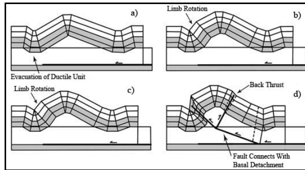
شکل ۸. توالی تکامل یک چین جدایشی گسل خورده. چین به صورت تقریباً متقارن شروع به تشکیل می‌کند (a و b) و تکامل آن به صورت نامتقارن، هم‌زمان با انتشار گسل است (c و d) [۷]
