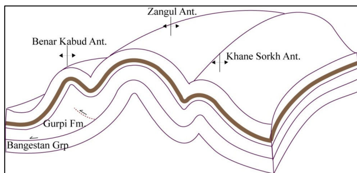
شکل ۴. بلوک دیاگرامی از تاقديس‌های فرعی در پهلوهای تاقديس زنگول
