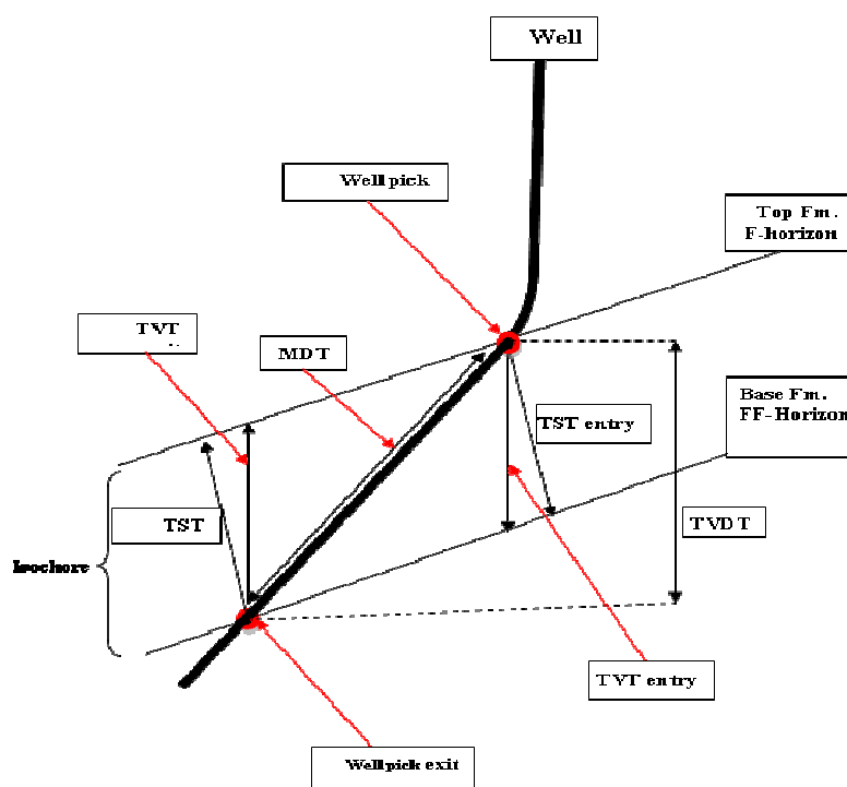
شکل ۲. روند محاسبه پارامترهای لازم در مدل سازی چینه ای
