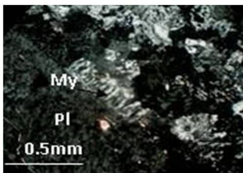
شکل ۵. بافت میرمکیت حاشیه‌ای
