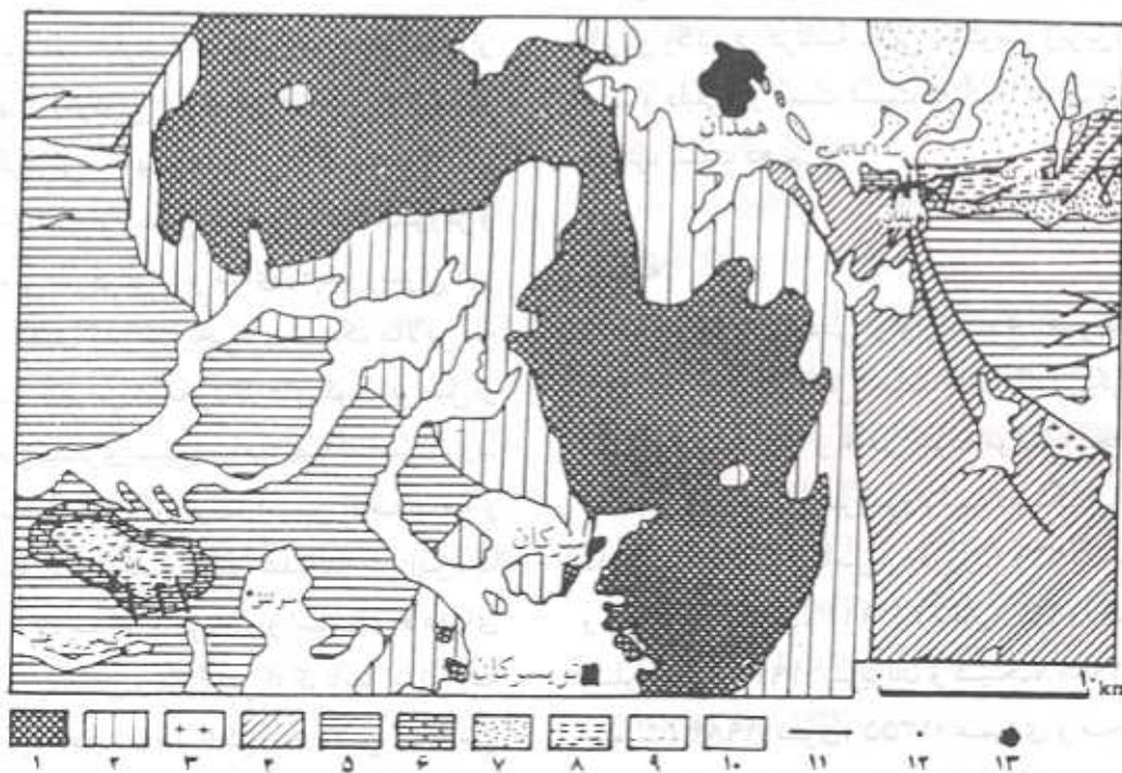
شکل ۱- نقشه زمین‌شناسی منطقه. ۱- نوده گرانیتوئید الوند، ۲- هورنفلس و هورنفلس شیت، ۳- پگماتیت، ۴- انواع شیت، ۵- اسلیت، ۶- آهک‌های ژوراسیک بالایی، ۷- ماسه‌سنگ کرتاسه، ۸- آهک و مارن کرتاسه، ۹- رسوبات میوسن، ۱۰- کواترنری، ۱۱- گل، ۱۲- روستا، ۱۳- شهر. (اقتباس با تغییراتی در چینه‌شناسی از نقشه زمین‌شناسی
