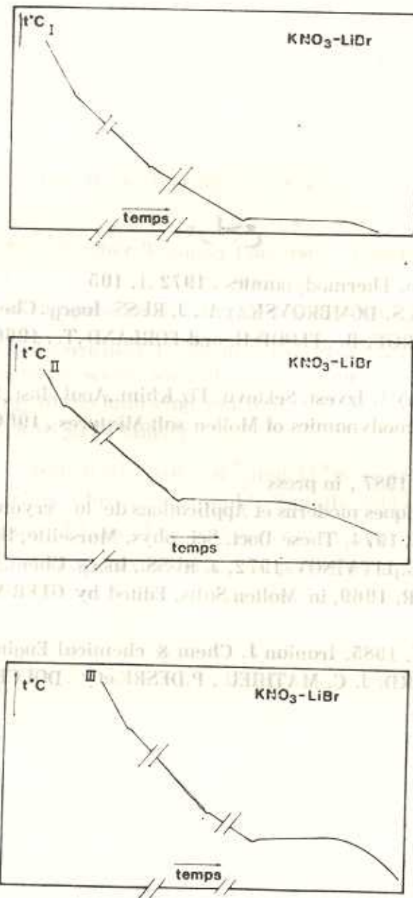
شکل ۴ منحنیهای دما - زمان در غلظتهای برای سیستم نیترات پتاسیم برمید لیتم
