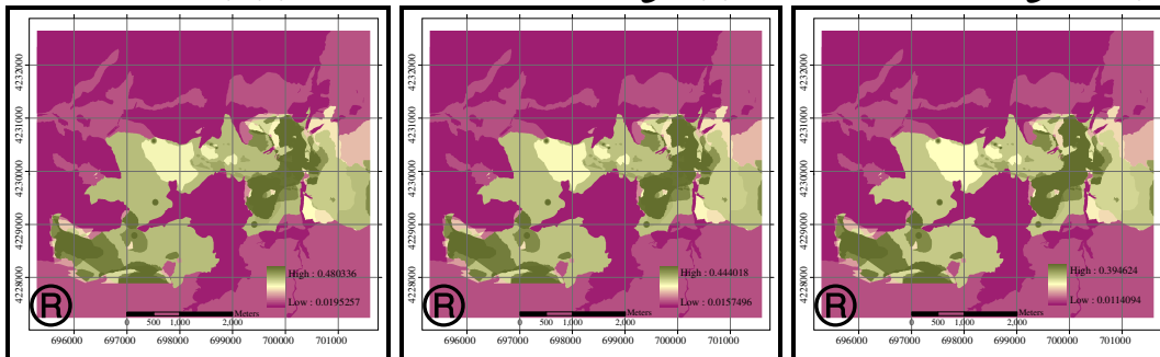
شکل ۱۶ - نقشه پتانسیل معدنی عملگر فازی \Gamma = 0.97
