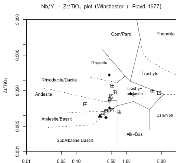
شکل ۶. نمودار Zr/TiO_2 در مقابل Nb/Y [۱۱]، بر مبنای این نمودار سنگهای آتشفشانی منطقه آستیان در قلمرو بازالت ساب آلکان، آندزیت بازالتی، آندزیت، تراکی آندزیت، داسیت، ریوداسیت و ریولیت قرار گرفته‌اند
