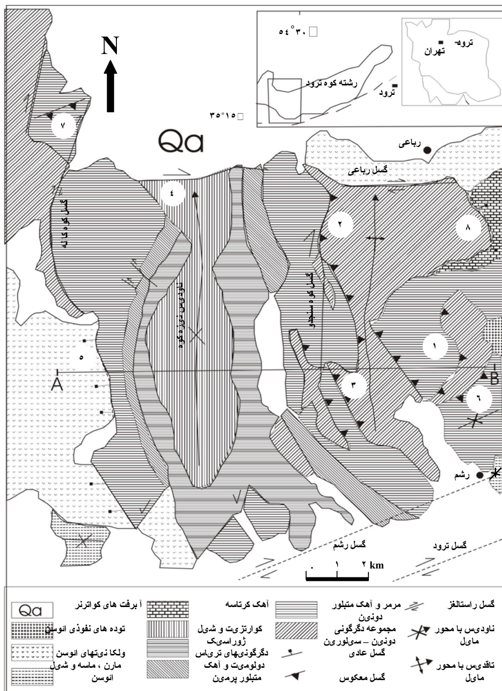
شکل ۱. نقشه زمین شناسی ساختمانی پایانه باختری گسل ترود (نقشه زمین شناسی پایه از هوشمند زاده و همکاران، ۱۳۵۷). برای توضیحات بیشتر ترود شرح اعداد به متن مراجعه شود.
