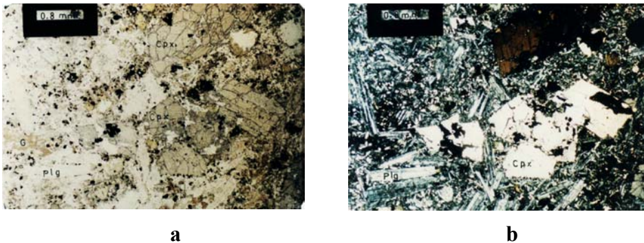
شکل ۱۱ - بازالت حاوی کلینوپیروکسن‌های اتومورف با ماکل ساعت شنی (بالا سمت راست) (Cpx)، پلاژیوکلاز (Plg)، کلریت (Cl) و شیشه (G) (سمت چپ و پایین) (۲۰x) (a) ppl (b) xpl
