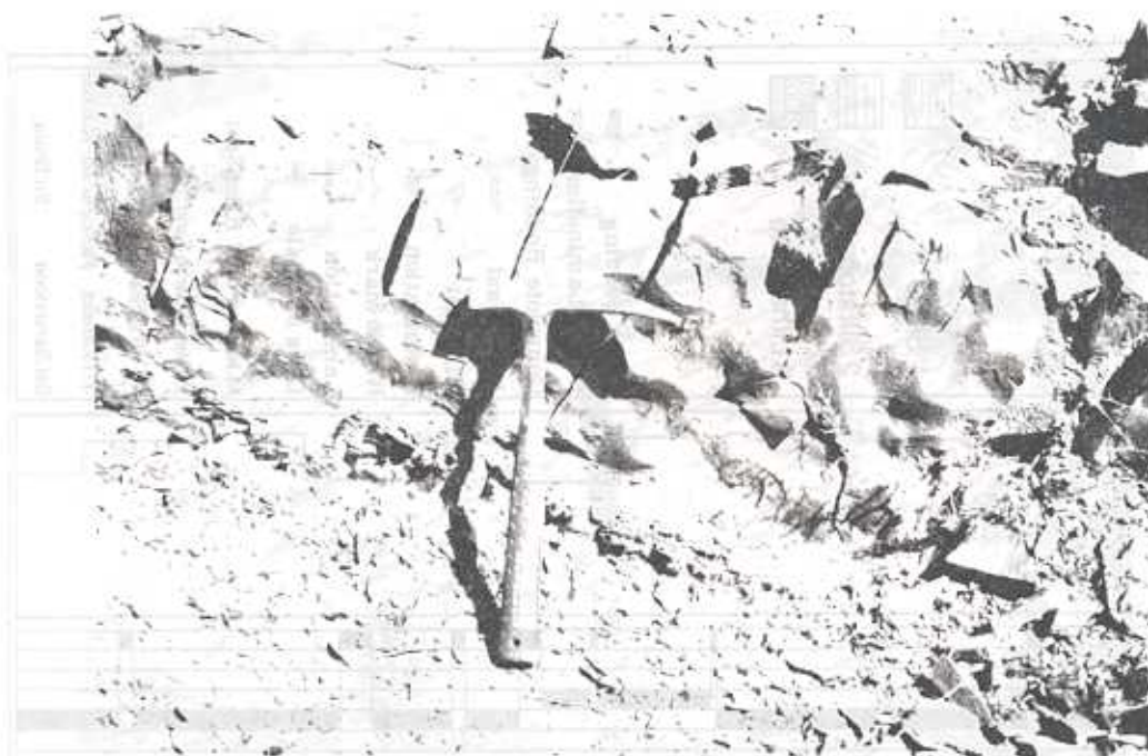
شکل ۹- دیبل مارک (جهت جریان از سمت چپ به سمت راست است).
