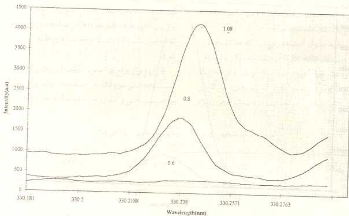
شکل ۳- اثر تغییرات توان پلازما بر حسب کیلووات بر روی شدت نشر محلول ۱۰ppmZn + ۳۰۰ ppmNa
