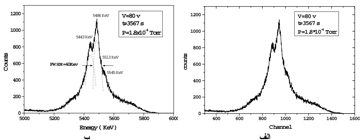
شکل ۲. الف) طیف ذرات آلفای ۵/۴۸ MeV از چشمه ^{241}\text{Am} آشکار شده با آشکارساز GaAs با تماس شاتکی دایره‌ای شکل به قطر ۳ mm و ضخامت ۴۰ μm، ب) طیف انرژی ذرات آشکار شده شکل ۲. الف
