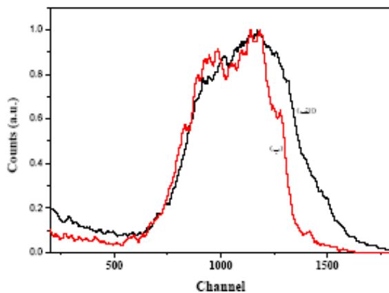
شکل ۵. طیف آلفای انداز گیری شده MeV\ 8/5 از چشمه ^{241}Am آشکار شده با آشکار ساز GaAs با تماس شاتکی دایره‌ای شکل به قطر 2\text{ mm} و ضخامت 400\ \mu\text{m} در ولتاژهای مختلف
