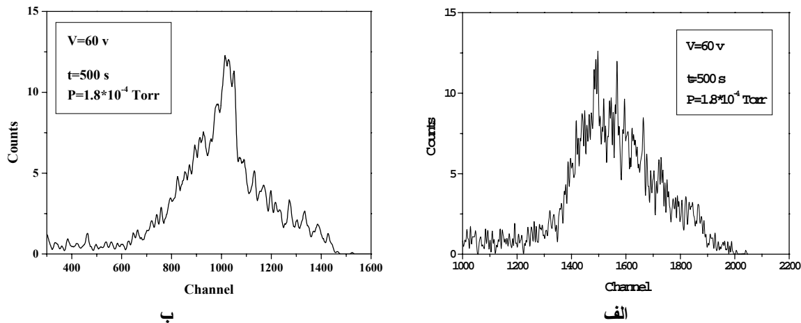
شکل ۳. طیف ذرات آلفای 5.48 \text{ MeV} از چشمه ^{241}\text{Am} آشکار شده با آشکار ساز \text{GaAs} با ضخامت 400 \mu\text{m} و تماس شاتکی دایره‌ای شکل به قطر: الف) ۱ mm ، ب) ۲ mm
