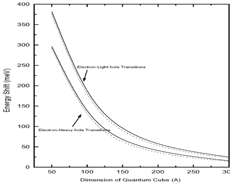
شکل ۲- جابه جایی انرژی حاملها در گذار الکترون- حفره سنگین و الکترون- حفره سبک بر حسب ابعاد نقاط کوانتومی سیستم GaAs / Ga_{0.63}Al_{0.37}As منحنی نقطه چین جابه جایی انرژی با در نظر گرفتن اثرات جرم در مرز و منحنی خط پر بدون در نظر گرفتن اثرات جرم مؤثر
