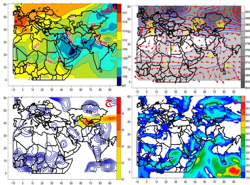
شکل ۵. الف) فشار سطح دریا به پاسکال (ب) ارتفاع ژئوپتانسیل تراز ۵۰۰ هکتوپاسکال به متر و جهت جریان باد تراز ۵۰۰ هکتوپاسکال به متر بر ثانیه (ج) امگا تراز ۵۰۰ به پاسکال و رودباد تراز ۲۵۰ هکتوپاسکال به متر بر ثانیه (د) رودخانه جوی کیلوگرم متر بر ثانیه
