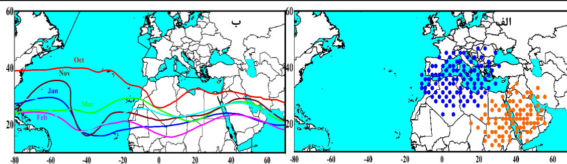
شکل ۴. موقعیت مکانی مراکز پرارتفاع جنب حاره عربستان و چرخندهای مدیترانه (الف) و موقعیت حد شمالی پرفشار جنب حاره (ب) در زمان خشکسالی‌های فراگیر کشور
