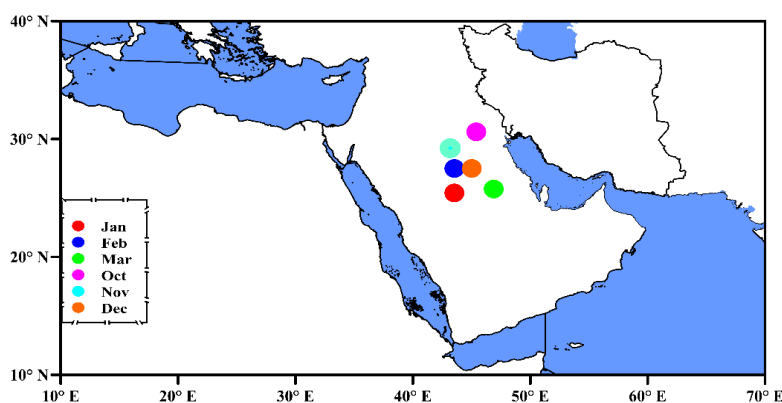
شکل ۸. موقعیت مراکز پشته پراتفیع عربستان در زمان خشکسالی ایران برای ماه‌های سرد سال
