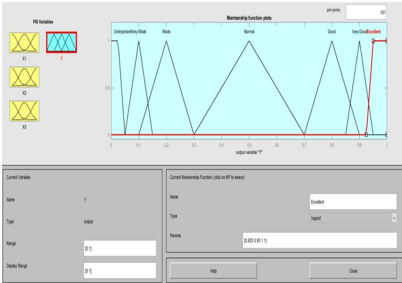
شکل ۵. افرارزبندی معیارها و تعیین مقادیر فازی مرتبط با متغیرهای زبانی (توابع عضویت اعداد مثلثی و ذوزنقه ای)
