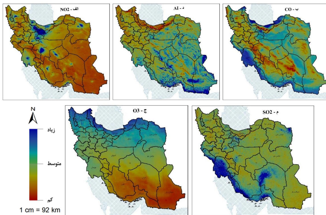
شکل ۸: کانون آلاینده‌های ایران در سال ۱۳۹۸، (الف) NO ۲ ، (ب) CO، (ج) O ۳ ، (د) AI، (م) SO ۲
