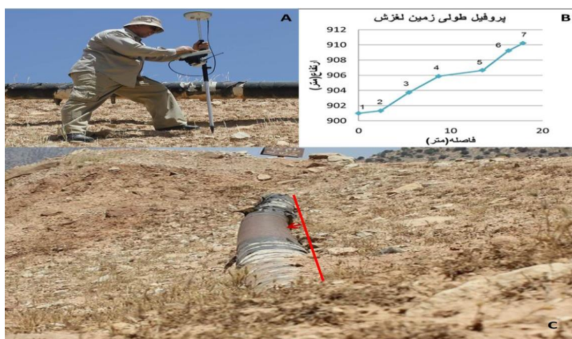
شکل ۱۲. عکس میدانی - پیمایش میدانی از زمین لغزش آسیب رسان به خط لوله حادث در مجاورت سد مارون (A) برداشت با دستگاه DGPS پروفیل ترسیمی از مقطع نمایش داده شده در شکل ۱۰ C نمای نزدیک از آسیب دیگی خط لوله انتقال گاز - خط قزمز به طول ۴ متر و پیکان واصل به میزان ۲۸ سانتیمتر خمیدگی لوله را نشان می‌دهد)
