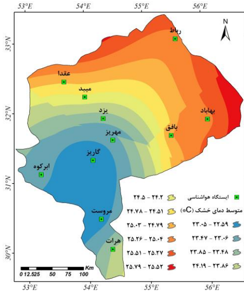
شکل ۱۳- توزیع فضایی میانگین دمای سالانه استان یزد طی روزهای گردوغباری / شکل ۱۴- توزیع فضایی متوسط دمای خشک استان یزد طی روزهای گردوغباری
