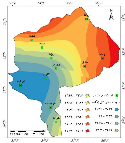
شکل ۱۳- توزیع فضایی میانگین دمای سالانه استان یزد طی روزهای گردوغباری / شکل ۱۴- توزیع فضایی متوسط دمای خشک استان یزد طی روزهای گردوغباری
