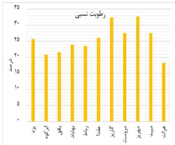
شکل ۱۵- متوسط رطوبت نسبی سالانه ایستگاه‌ها طی روزهای گردوغباری / شکل ۱۶- توزیع فضایی متوسط رطوبت نسبی سالانه استان یزد طی روزهای گردوغباری
