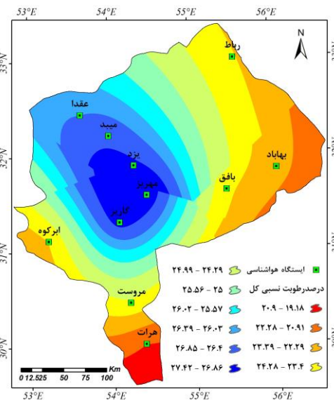
شکل ۱۵- متوسط رطوبت نسبی سالانه ایستگاه‌ها طی روزهای گردوغباری / شکل ۱۶- توزیع فضایی متوسط رطوبت نسبی سالانه استان یزد طی روزهای گردوغباری
