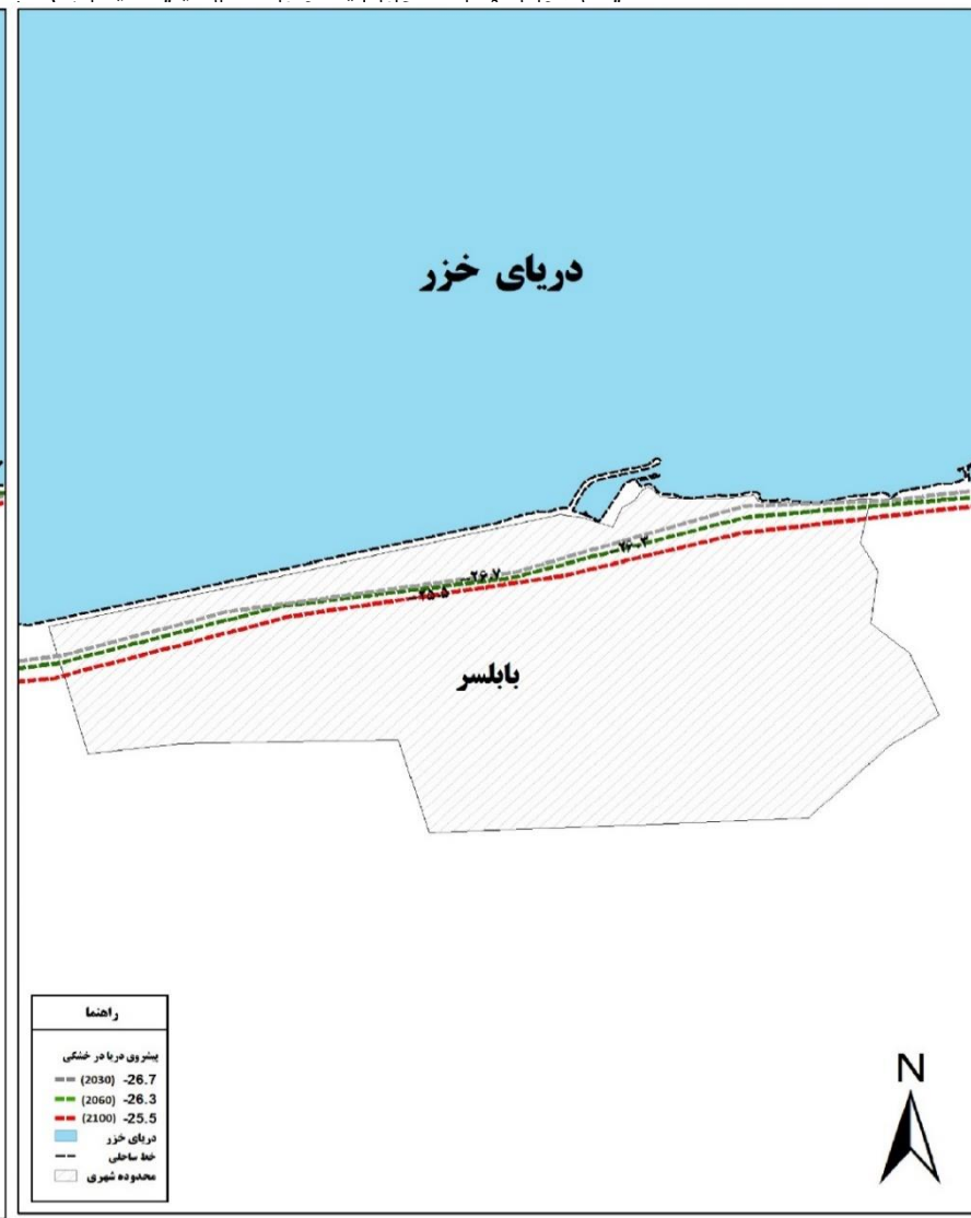
شکل ۱۸: پیش بینی محدوده عقب نشینی خط ساحلی بابلسر در سناریوی RCP 4.5 و RCP 8.5
