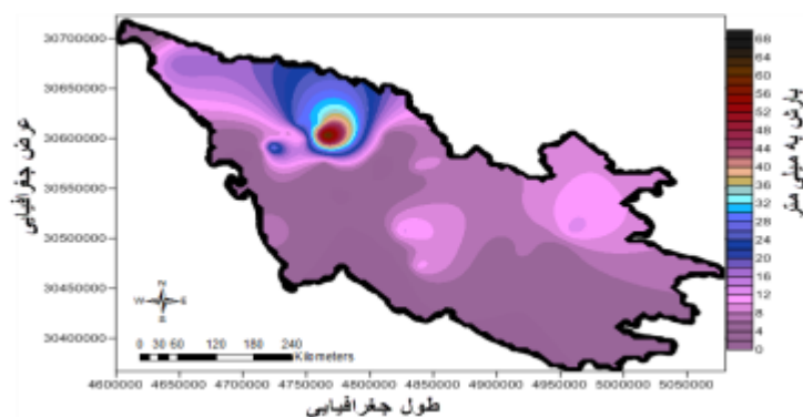
شکل ۲۰: نقشه پهنه‌بندی بارش سنگین در روز ۲۴ مارس ۱۹۹۶
