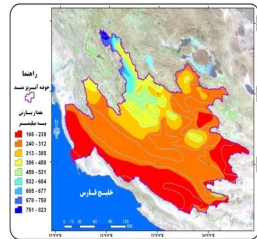
شکل ۶: پهینه‌بندی بارش در محدوده‌ی مطالعه.
