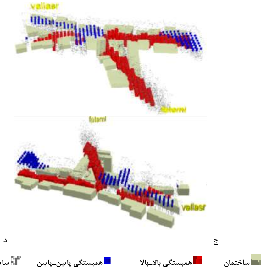
شکل ۱۲: شمایی سه بعدی از نحوه پراکنش غلظت آلاینده NO_x در ارتفاعات مدل سازی شده از نماهای متفاوت.
