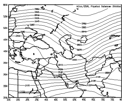
شکل ۱۶. الگوی سینوپتیکی حاکم در تراز ۷۰۰ هکتوپاسکال در روز همراه با بارش برف (الگوی CP۴)
