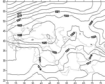
شکل ۱۴. الگوی سینوپتیکی حاکم در تراز سطح دریا در روز همراه با بارش برف (الگوی CP۴)
