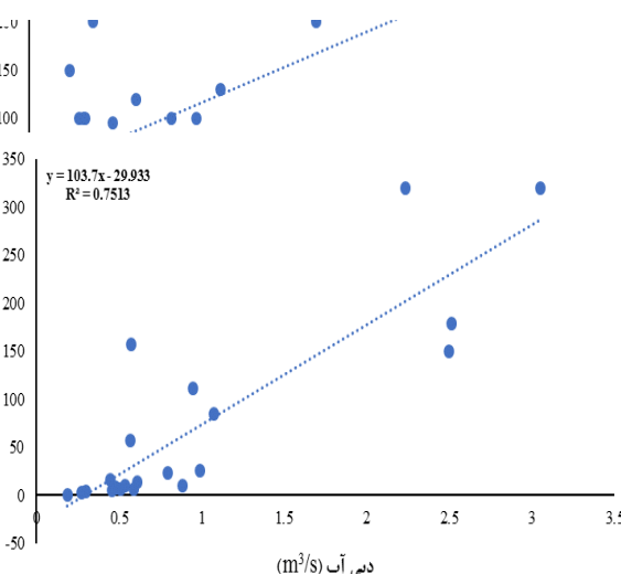
شکل ۱۴. منحنی سنج رسوب سالانه ایستگاه سفیدچاه
