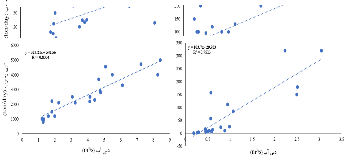
شکل ۱۳. منحنی سنج رسوب سالانه ایستگاه آیلو
