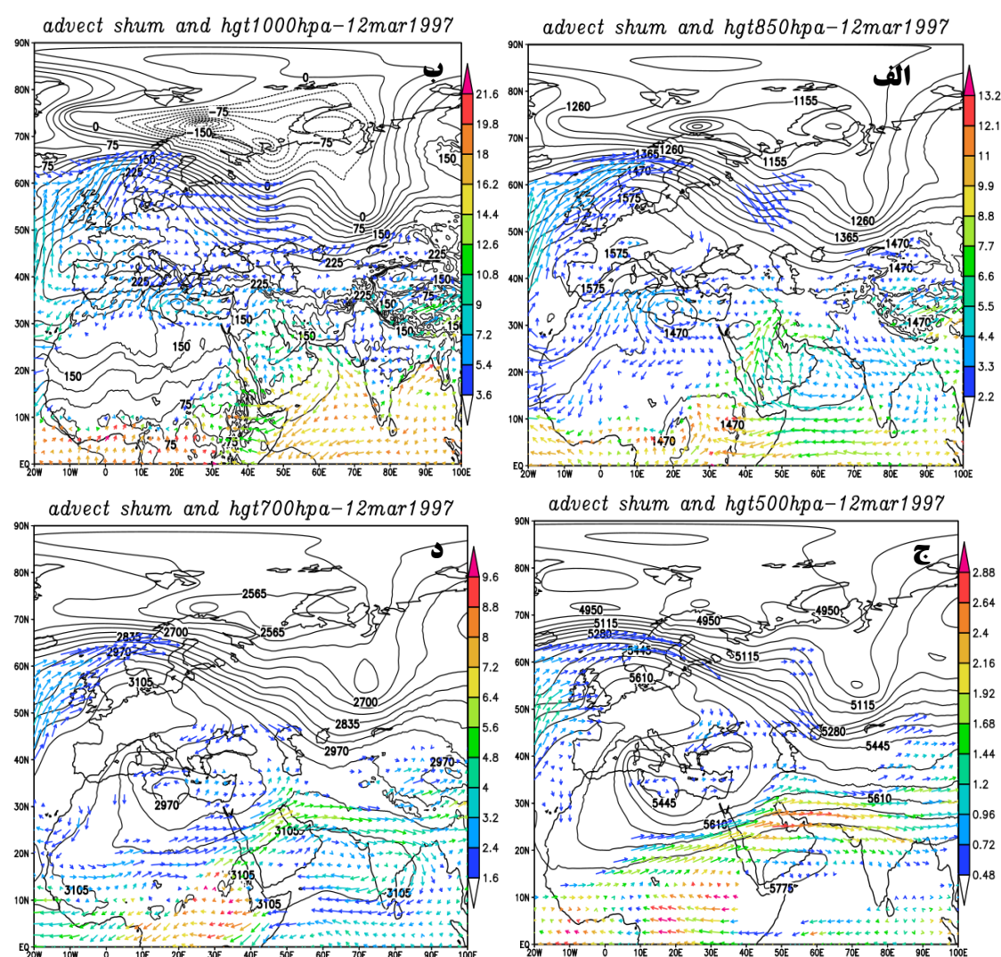
شکل ۱۹. نقشه های ترکیبی ارتفاع ژئوپتانسیل و وزش رطوبتی ترازهای ۱۰۰۰ تا ۵۰۰ هکتوپاسکال الگوی چهارم در روز نماینده ۱۲ مارس ۱۹۹۷
