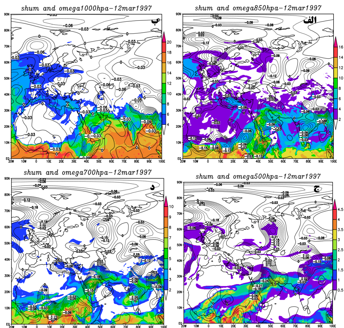
شکل ۲۰. نقشه های ترکیبی نم و ویژه و امگای ترازهای ۱۰۰۰ تا ۵۰۰ هکتوپاسکال الگوی چهارم در روز نماینده ۱۲ مارس ۱۹۹۷
