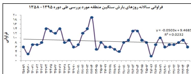
شکل ۴. روند فراوانی سالانه روزهای بارش سنگین منطقه مورد مطالعه طی دوره ۱۳۵۸-۱۳۹۵
