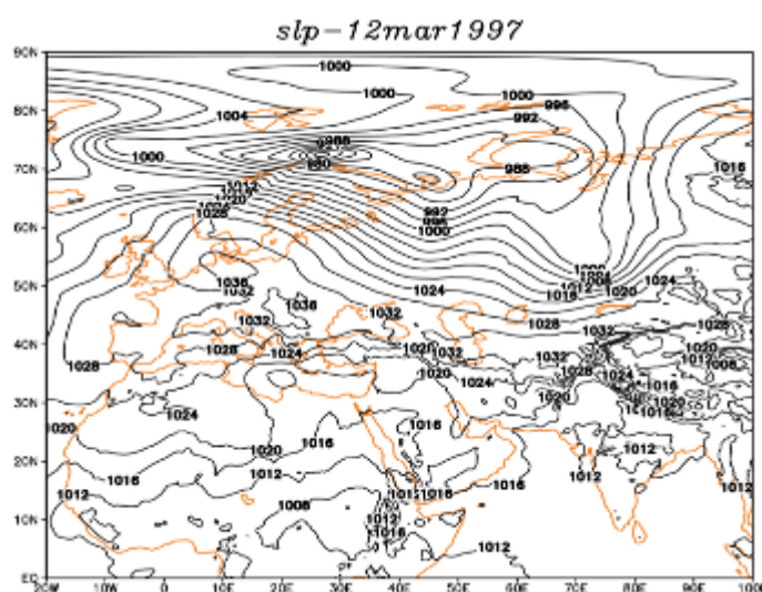
شکل ۱۸. نقشه فشار تراز دریای الگوی چهارم در روز نماینده ۱۲ مارس ۱۹۹۷
