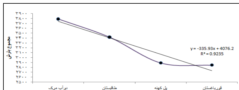
شکل ۲. مجموع بارش ایستگاههای مورد بررسی طی دوره ۱۳۵۸-۱۳۹۵
