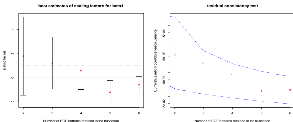
شکل ۴: شکل چپ (ج) میانه و محدوده اطمینان ۹۰٪ ضرایب مقیاس ساز ( \beta ) در EOF های مختلف برای متوسط بارش زمستانه تحت سیگنال GHG، شکل راست (ح) نتایج آزمون ثبات باقیمانده های EOF های متناظر و دامنه ۵-۹۵ درصد عدم قطعیت آزمون
