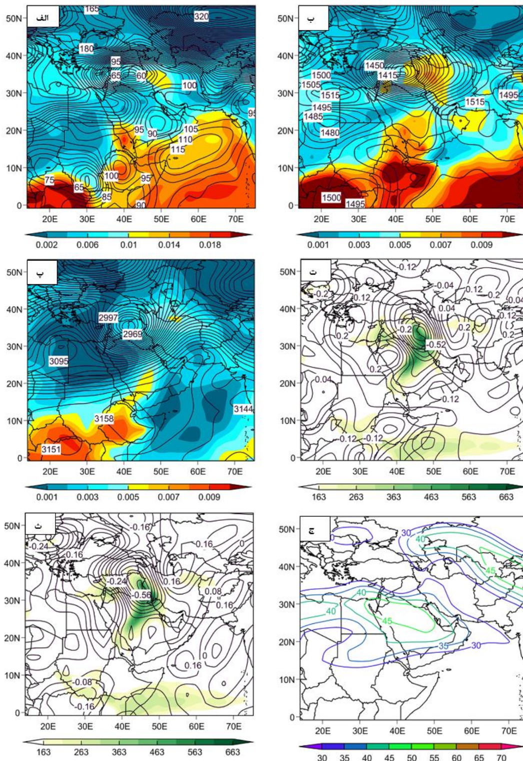
شکل ۱۳. الف) نقشه ترکیبی ژئوپتانسیل متر و نم ویژه به کیلوگرم در کیلوگرم روز ۱۸ فوریه ۲۰۱۸ (تراز ۱۰۰۰، ب) تراز ۸۵۰ و پ) تراز ۷۰۰ هکتوپاسکال، ت) نقشه ترکیبی رودخانه (IVT) در ساعت اوج به همراه امگای تراز ۷۰۰ (ت) و تراز ۵۰۰ هکتوپاسکال، ج) نقشه جت تراز ۲۵۰ هکتوپاسکال
