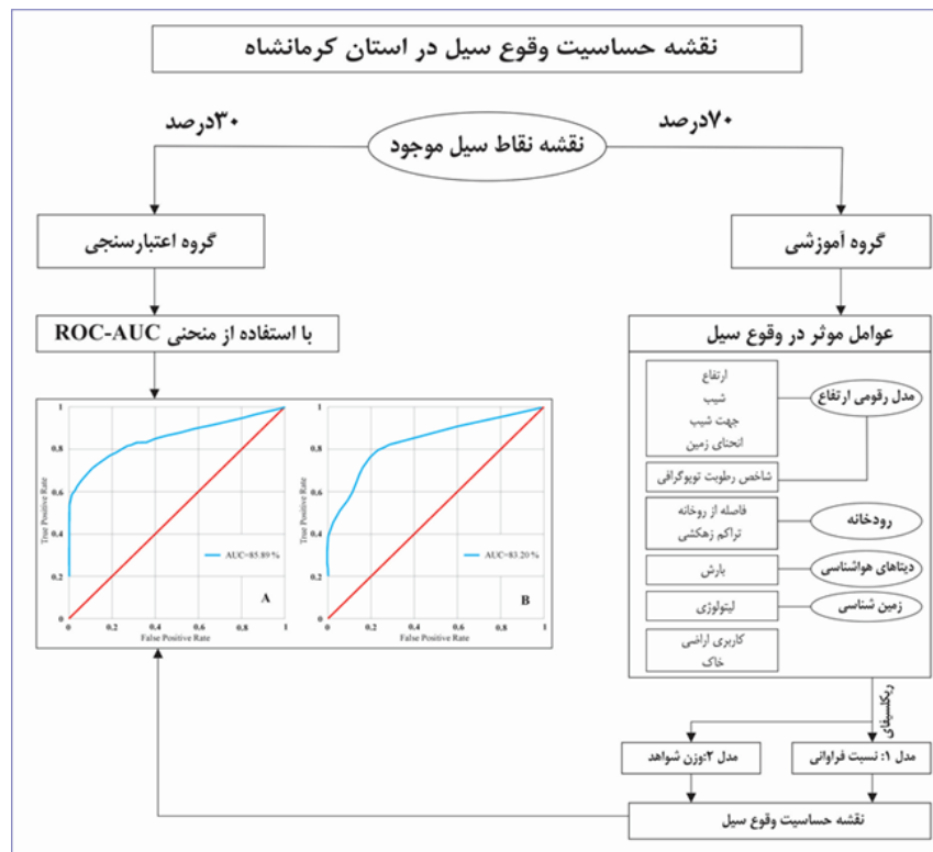
شکل ۲. نمودار جریان‌ی روند پردازش داده‌ها در تهیه نقشه حساسیت سیل در این مطالعه
