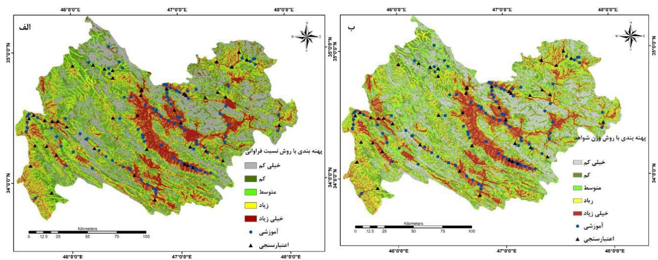
شکل ۴. پهنه‌بندی خطر حساسیت سیل استان کرمانشاه: الف: مدل نسبت فراوانی FR، ب: مدل وزن شواهد WofE
