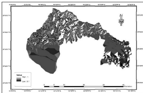
شکل ۸. فازی سازی طبقات جهت شیب.
