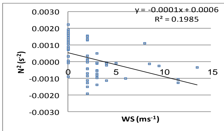
شکل ۵. نمودار پراکنندگی پایداری جو ( N^2 ) و تندی باد (WS) در ژانویه ۲۰۰۷.
