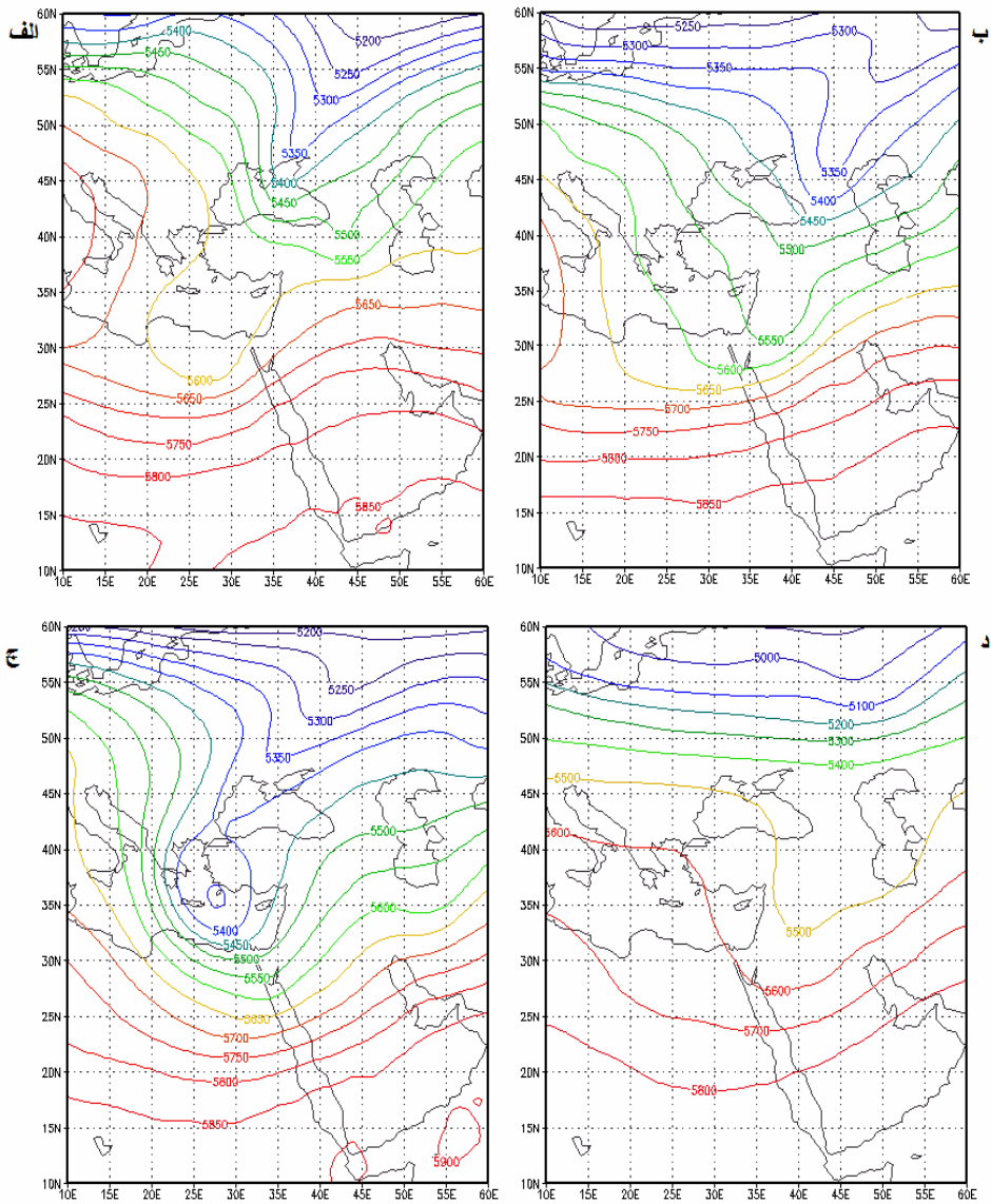
شکل (۱) مکان گزینی ناوه سامانه ترکیبی مدیترانه‌ای- سودانی در ساعات مختلف تراز ۵۰۰ هکتوپاسکال، (الف) ساعت ۰۰ utc روز ۴ فوریه ۱۹۹۵ (ب) ساعت ۱۸ utc روز ۴ فوریه ۱۹۹۵ (ج) ساعت ۱۸ utc روز ۶ فوریه ۱۹۹۵ (د) ساعت ۱۸ utc روز ۸ فوریه ۱۹۹۵
